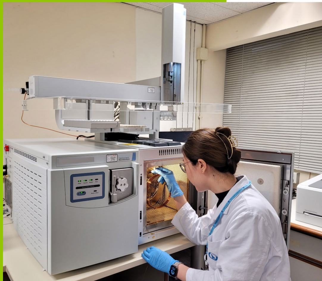
利用气相色谱串联质谱联用仪分析挥发性有机化合物
