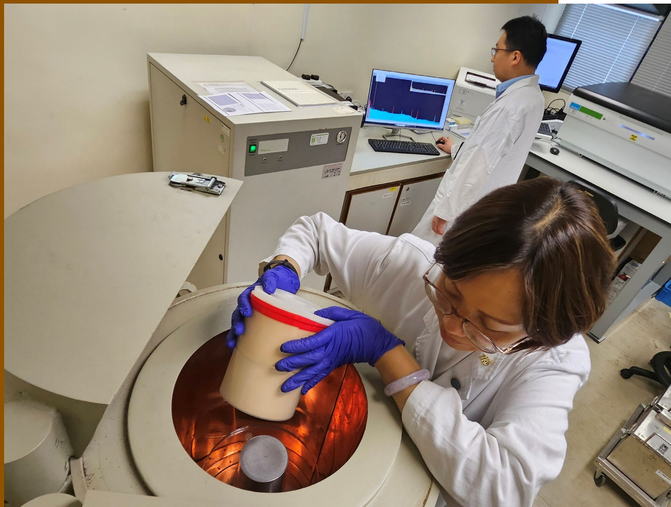
用于分析食物中放射性核素的伽玛能谱仪系统
