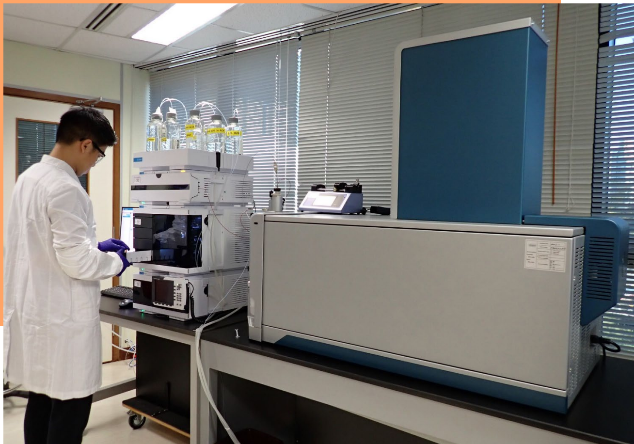
使用高效液相层析串联飞行时间质谱仪为生物样本进行药物及毒品筛查
