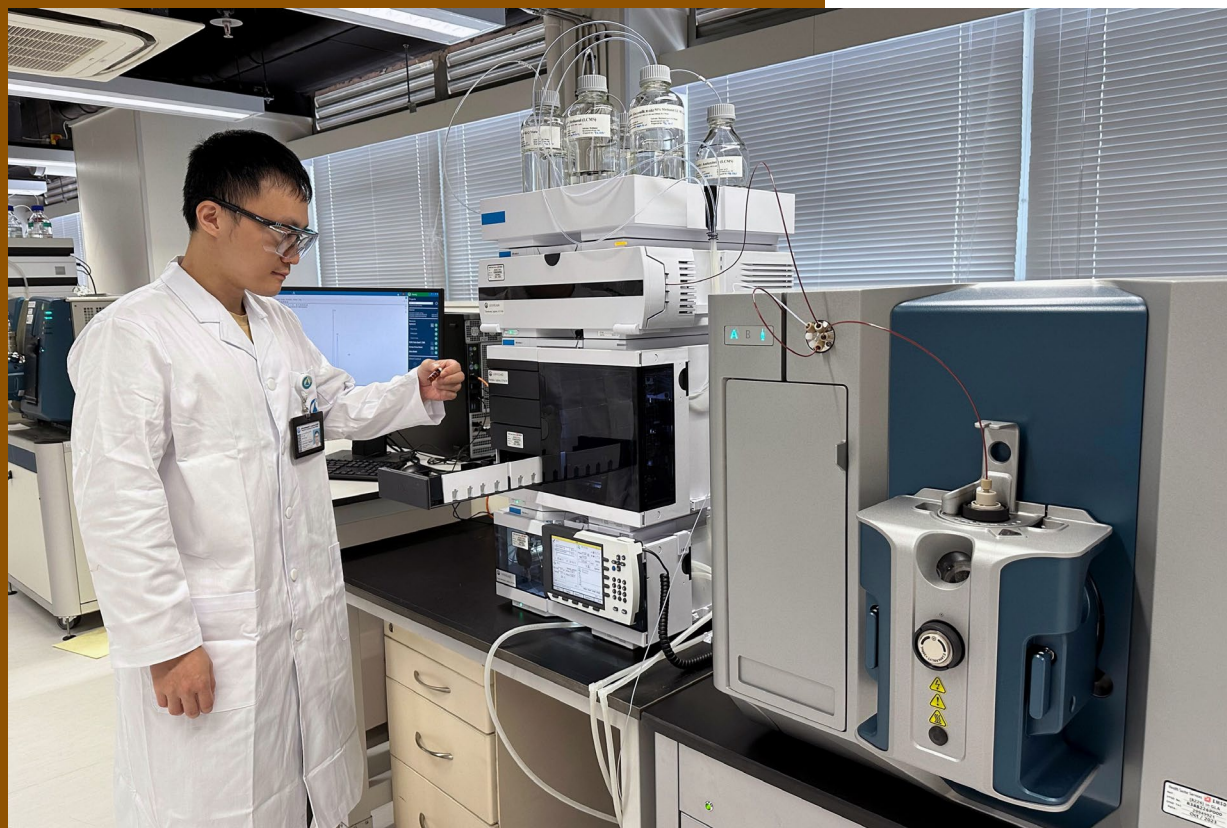
用作食物营养标签中相关检测的液相色谱串联质谱联用仪
