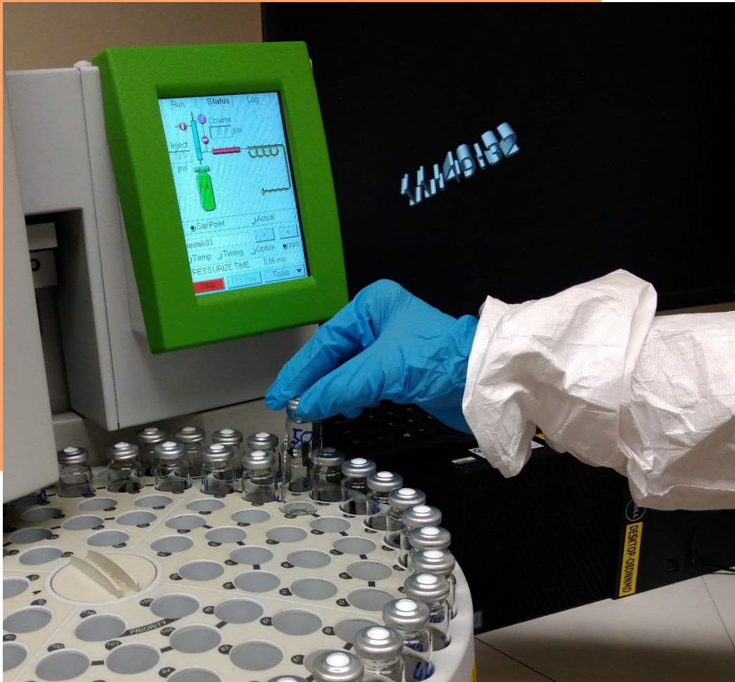
使用顶空气相色谱分析血液酒精含量
