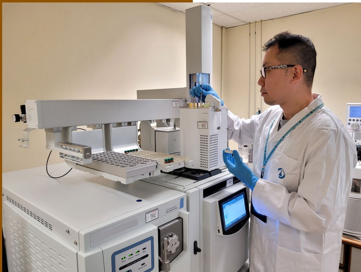
使用新购置的热解气相色谱串联质谱联用仪进行实验
